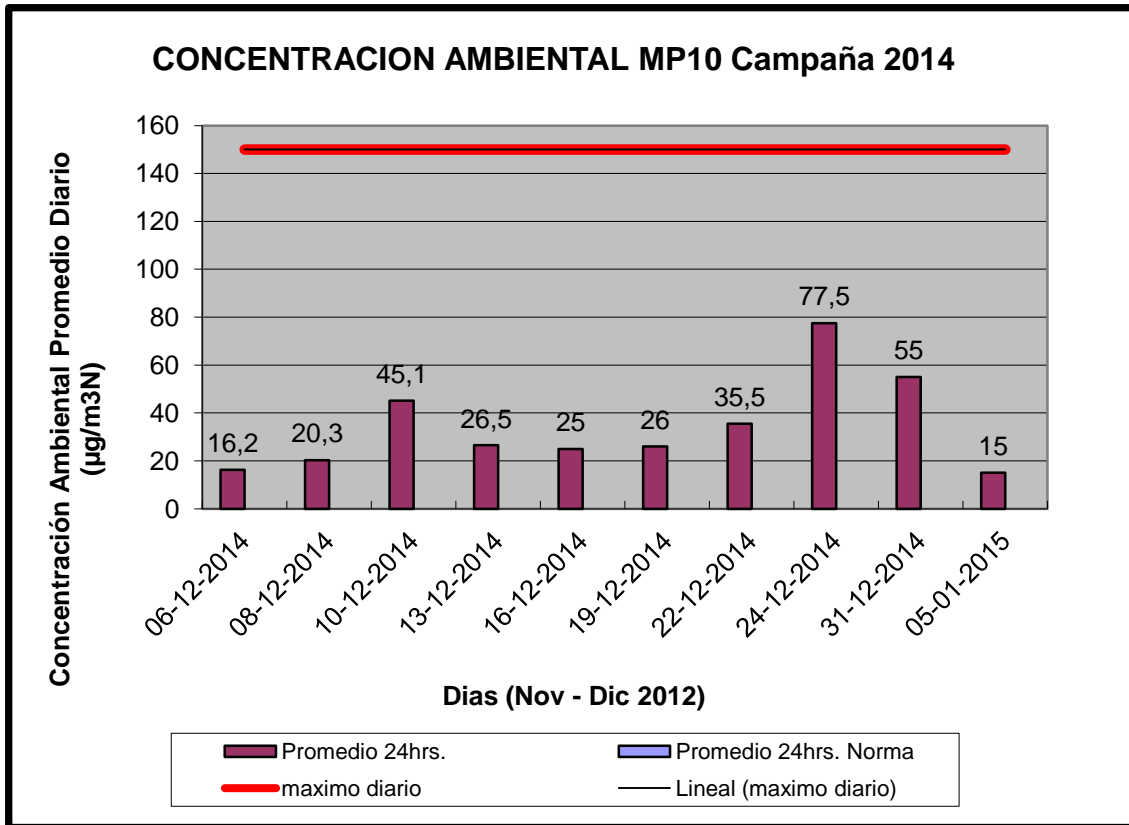
Gráfico N° 6: Concentraciones ambientales periodo 2014
