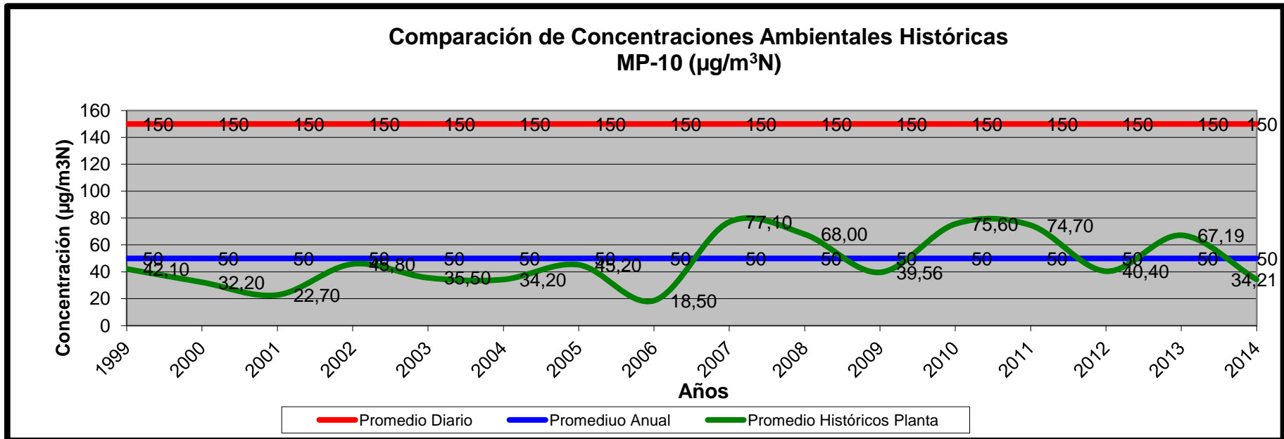
Gráfico N° 3: Concentraciones Históricas de Material Particulado
