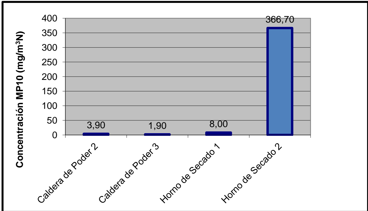
Gráfico N° 5: Emisiones Totales Complejo periodo 2014
