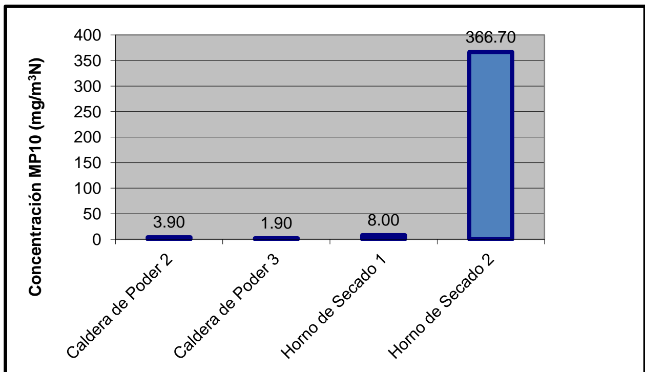
Gráfico N° 1: Emisiones de Material Particulado Complejo, expresado como Concentración
