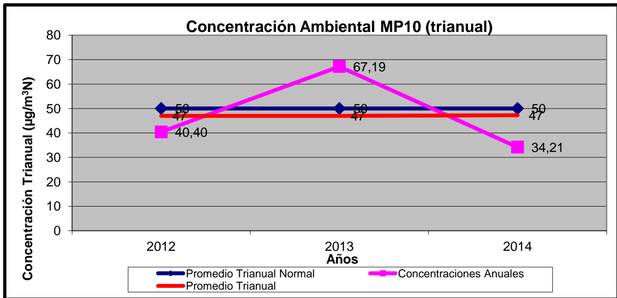
Gráfico N° 4: Concentraciones Trianuales de Material Particulado
