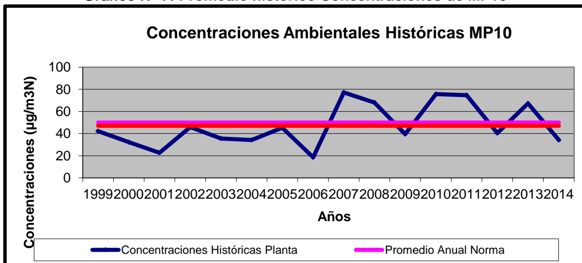
Gráfico N° 7: Promedio histórico Concentraciones de MP10
