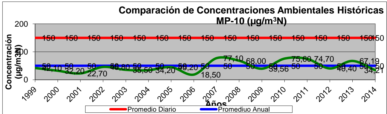
Gráfico N° 8: Concentraciones históricas de MP10
