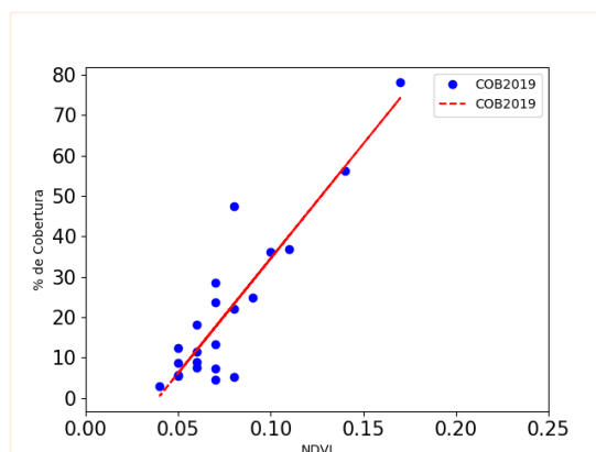
Figura 2-2. Relación de porcentaje de cobertura de vegetal obtenida en terreno mediante transectos y valores medios de NDVI obtenidos del análisis de imágenes. Borde Este del Salar de Atacama.
