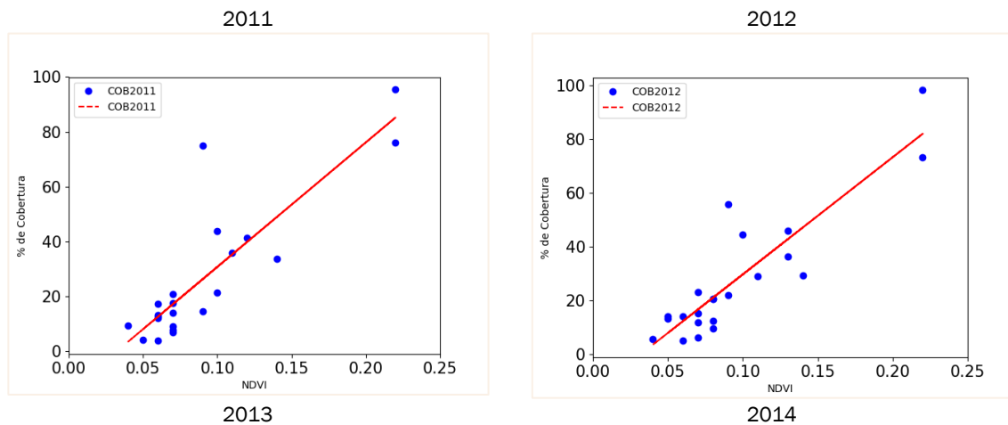
Figura 2-2. Relación de porcentaje de cobertura de vegetal obtenida en terreno mediante transectos y valores medios de NDVI obtenidos del análisis de imágenes. Borde Este del Salar de Atacama.
