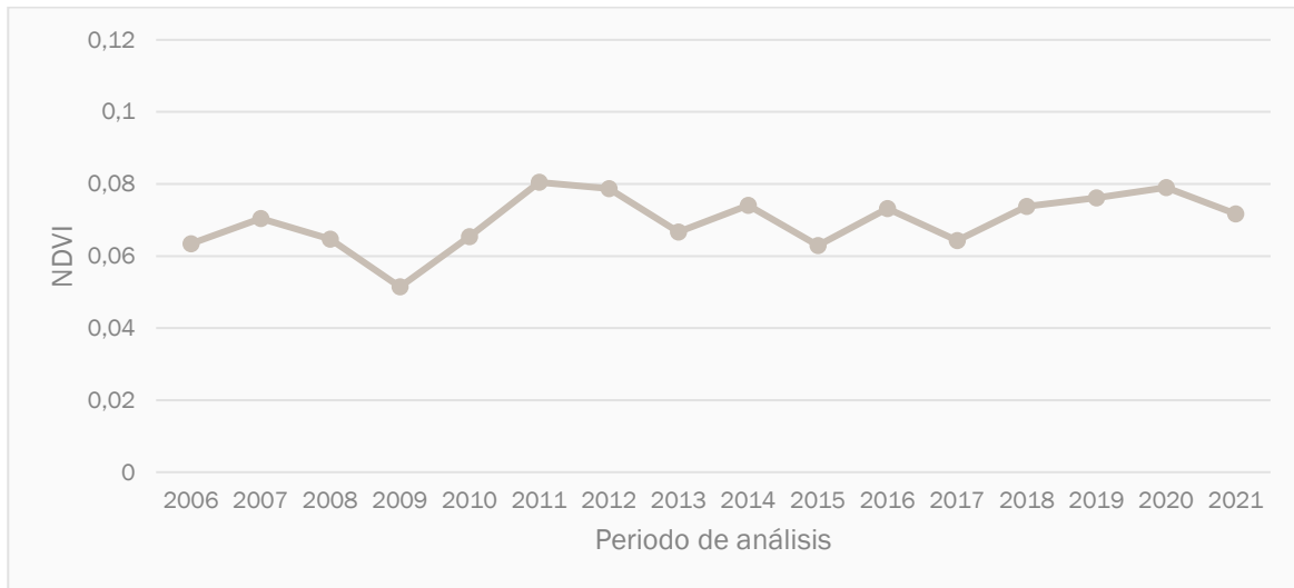
Figura 3-1. Promedio de los valores NDVI del área cubierta con vegetación en el Borde Este del Salar de Atacama en el periodo operacional (2006 – 2021)
