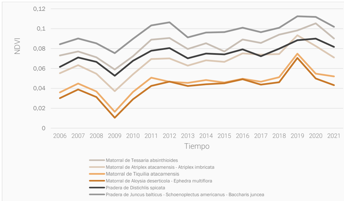
Figura 3-3. Valores promedios NDVI de unidades con tendencia al alza para cada tipo vegetacional en el Periodo Operacional (2006-2021)
