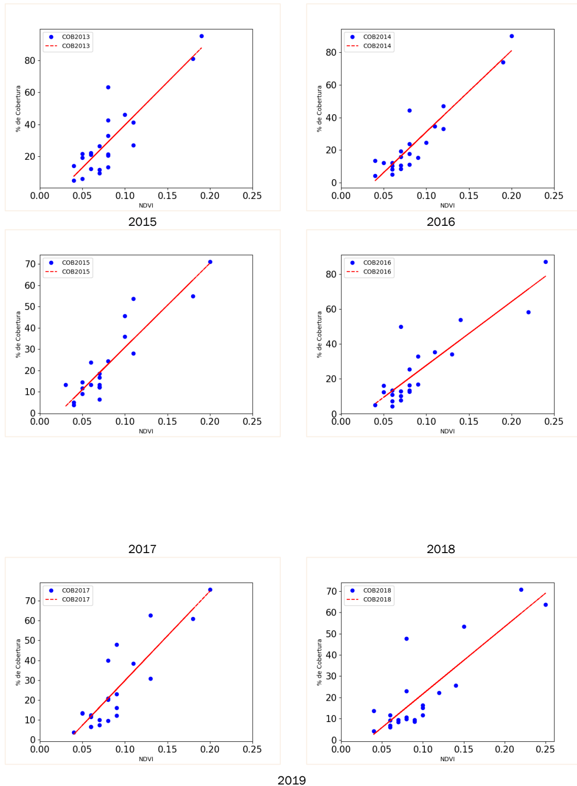
Figura 2-2. Relación de porcentaje de cobertura de vegetal obtenida en terreno mediante transectos y valores medios de NDVI obtenidos del análisis de imágenes. Borde Este del Salar de Atacama.
