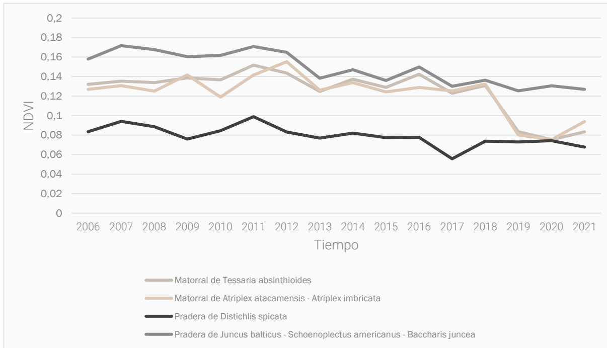
Figura 3-2. Valores promedio NDVI de unidades con tendencia a la baja para cada tipo vegetacional en el periodo operacional (2006-2021)
